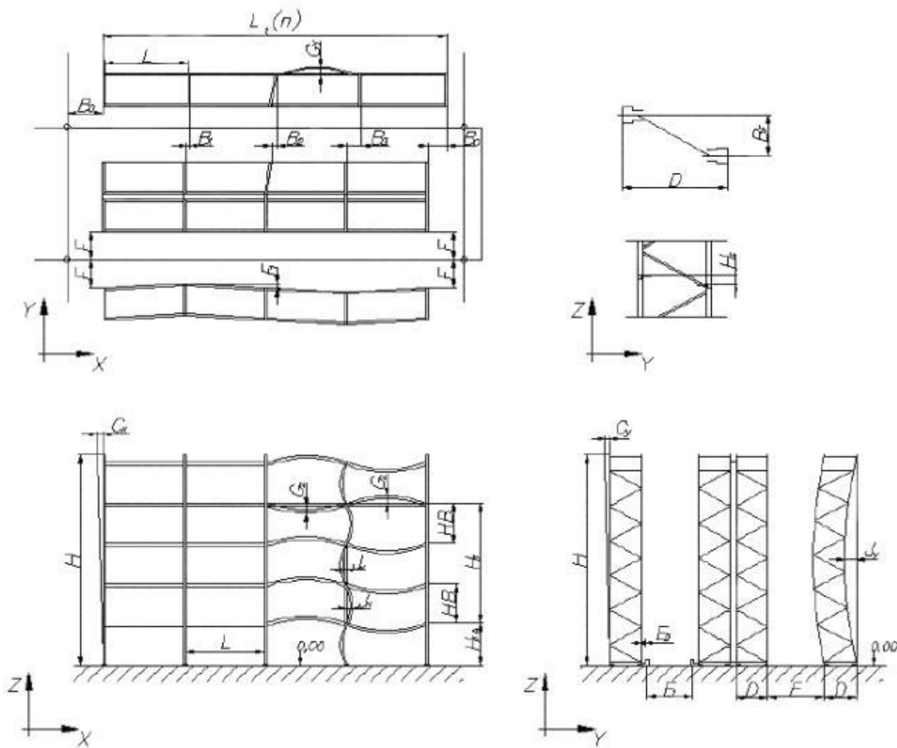
Рисунок 7 - Параметры, подлежащие контролю в ненагруженном состоянии системы
