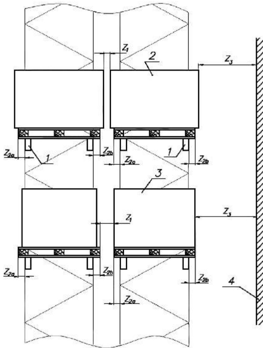
1 - балка; 2 - поддон со свесом груза; 3 - поддон без свеса груза; 4 - стена здания, коммуникации, либо другие, не относящиеся к стеллажам, объекты; Z_1 - минимальное из двух расстояний: между грузами, либо между поддонами; Z_2 (Z_{2a}, Z_{2b}) - свес поддона относительно балок (левой и правой); Z_3 - расстояние до стен здания, коммуникаций, а также других объектов
