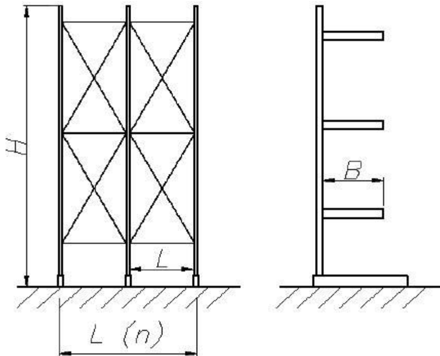
Рисунок 3 - Общий вид консольного стеллажа
